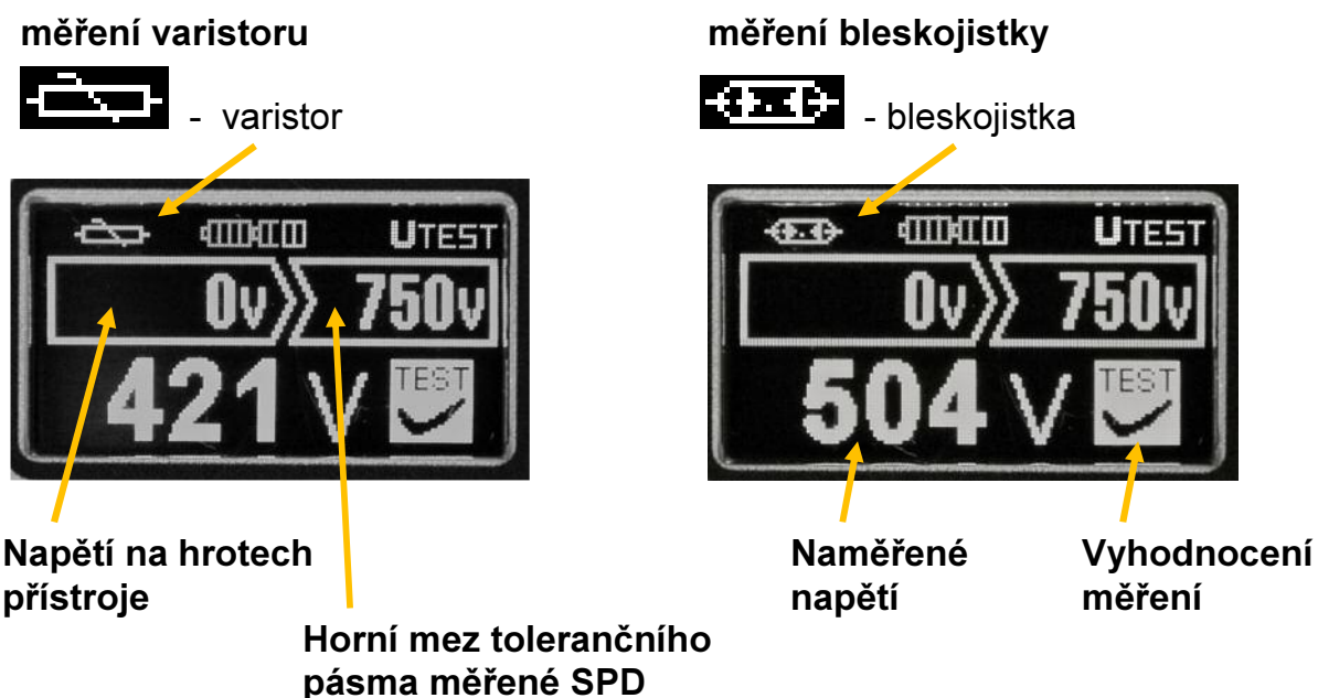
Obr. 3.9 Příklad zobrazení výsledku měření vybrané SPD na displeji přístroje
