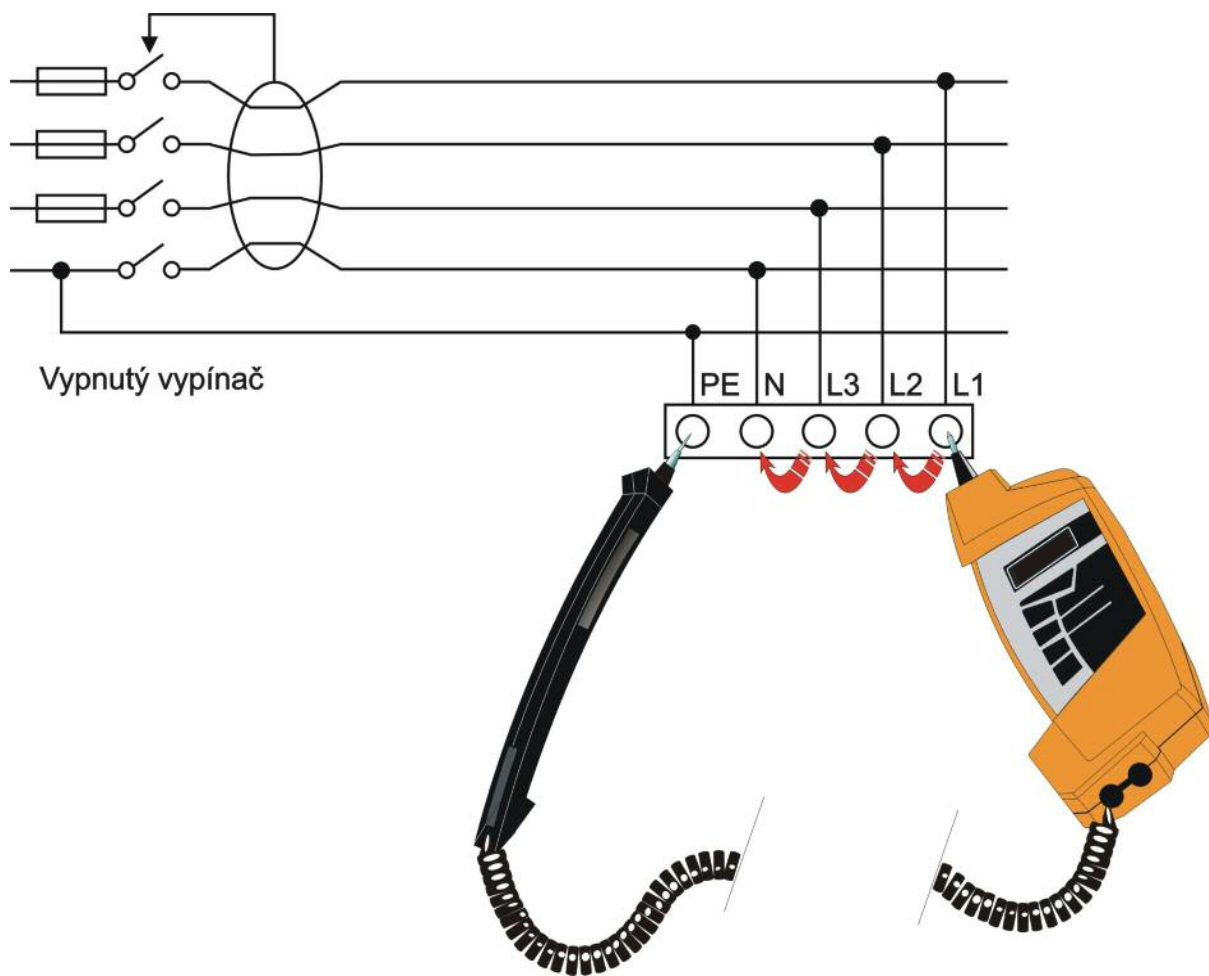
Obr. 3.6 Příklad zapojení
