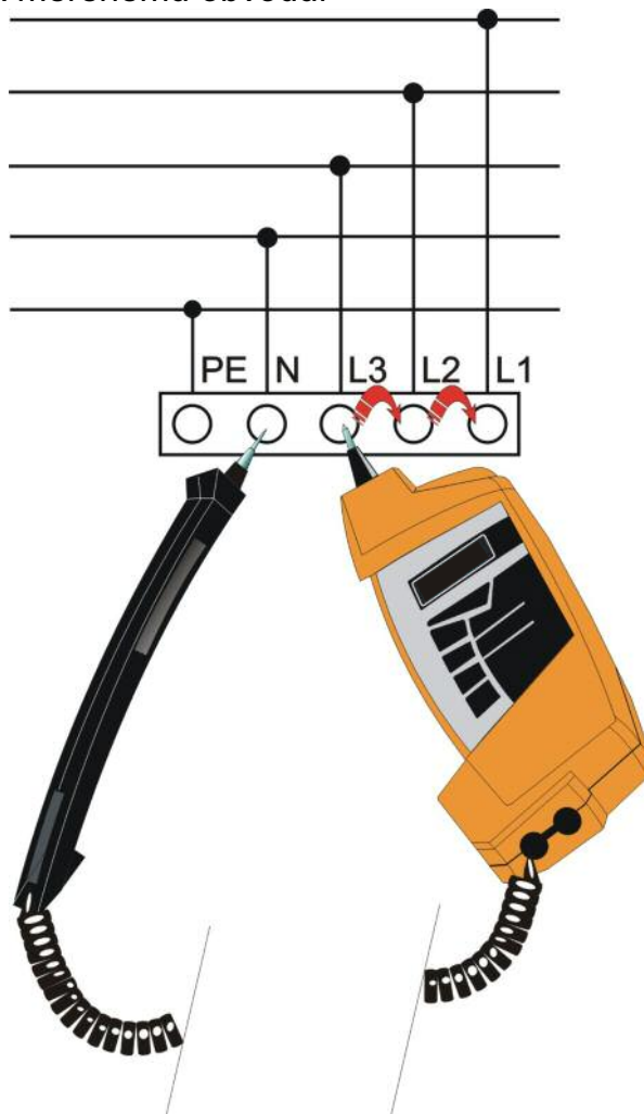
Obr. 3.3 Příklad zapojení
