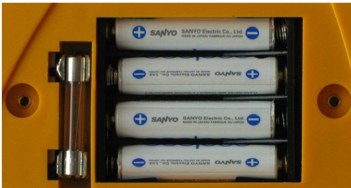
Obr. 4.1 Správná polarita napájecích článků a umístění pojistky
