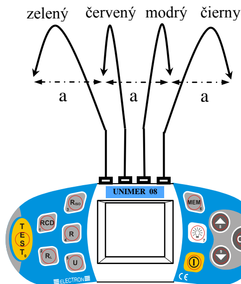
Obr. 4: Pripojenie sond pri meraní špecifického zemného odporu
