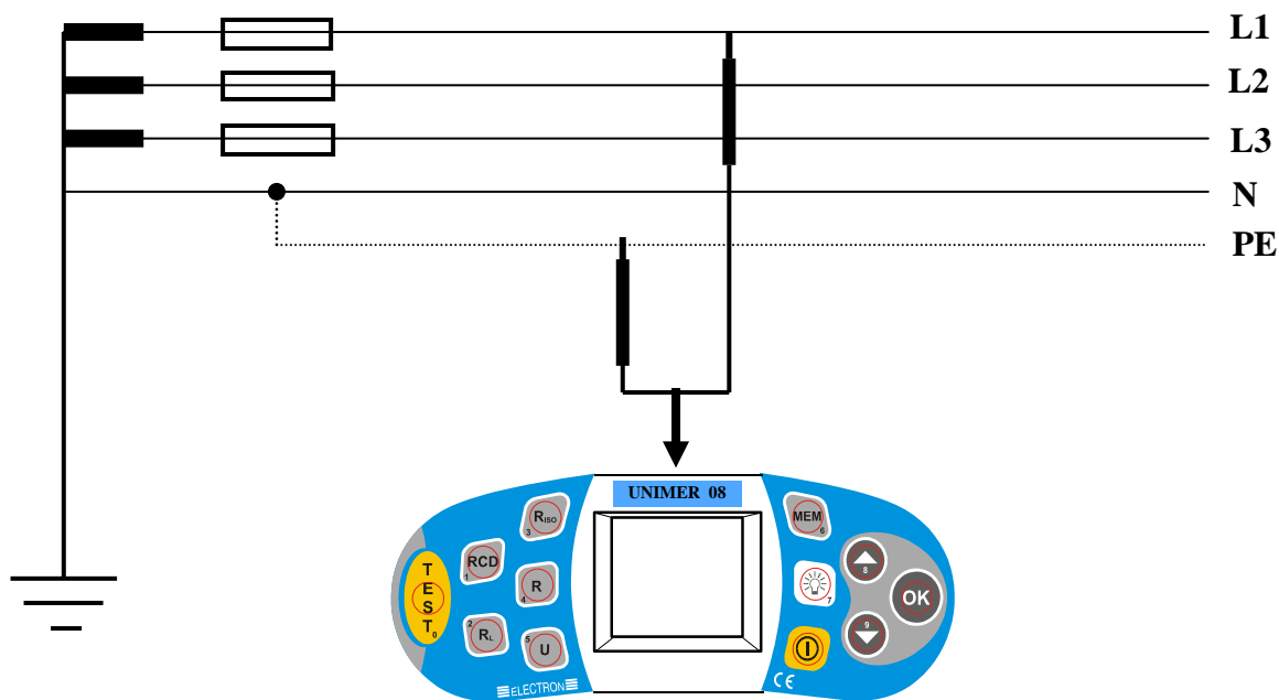
Obr. 1: Meranie impedancie pomocou prívodu pre dvojpólové meranie
