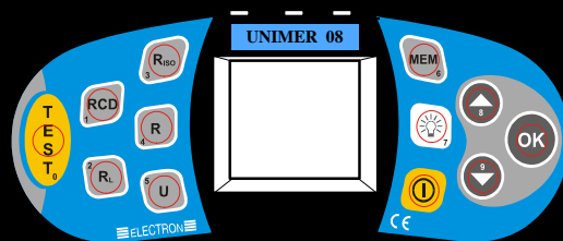
Obr. 3: Meranie zemných odporov pomocou sond
